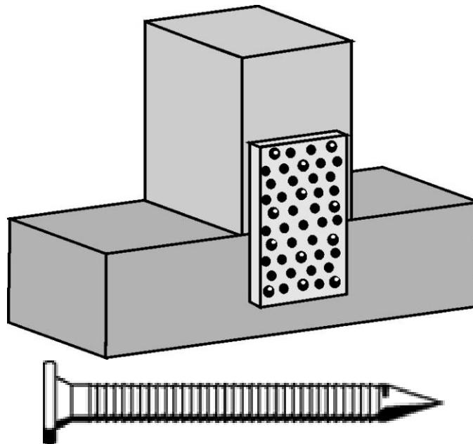
Kammnagel
